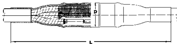
Wymiary L, D – w tablicy obok
