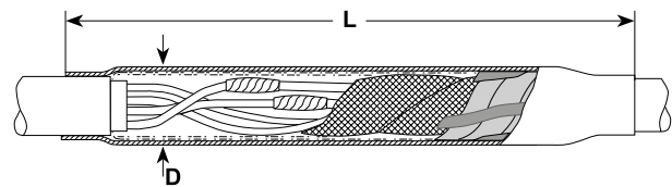
Wymiary L, D patrz tablica poniżej
